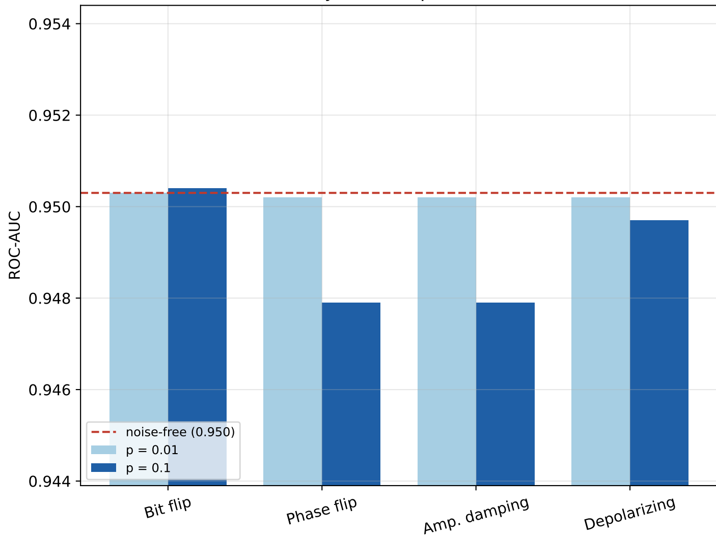
PaySim (comparison)
